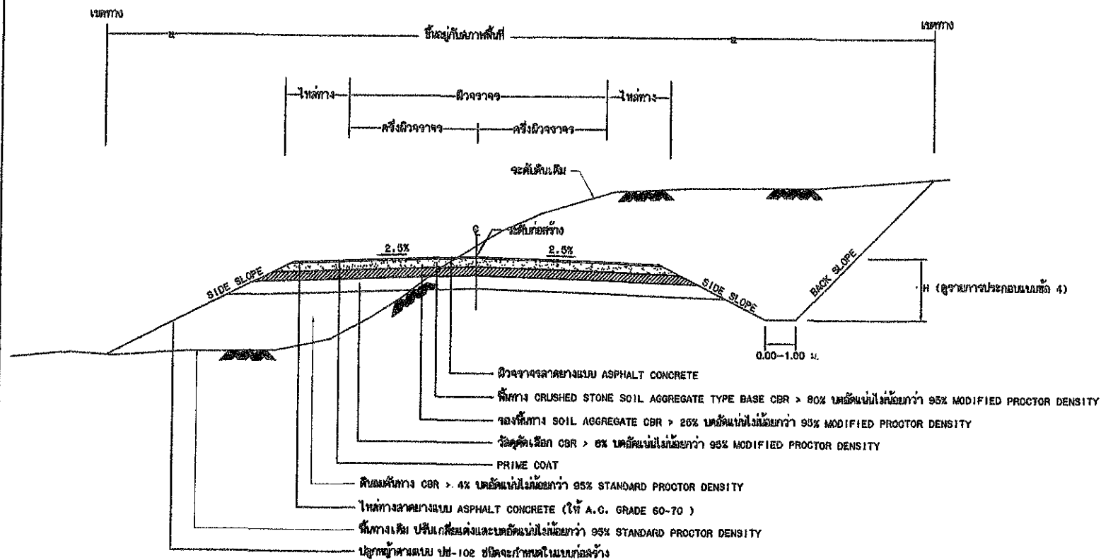
รูปตัดและผังโครงสร้างถนนดินตัด ดินถมและคลุมทับด้วยวัสดุ
