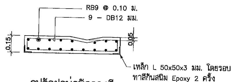
รูปตัดผาบ่อพิภรางวี (การเสริมเหล็กต่อ 1 ผา)
