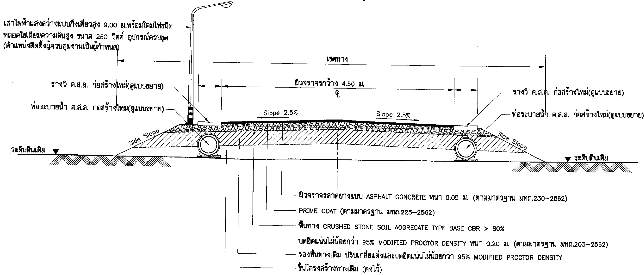
รูปตัดแสดงโครงสร้างถนนและคุณสมบัติวัสดุ (รูปตัดแสดงโครงสร้างชั้นทางเท่านั้น) (ช่วงที่ 1 Sta.0+150-Sta.0+242) NOT TO SCALE
