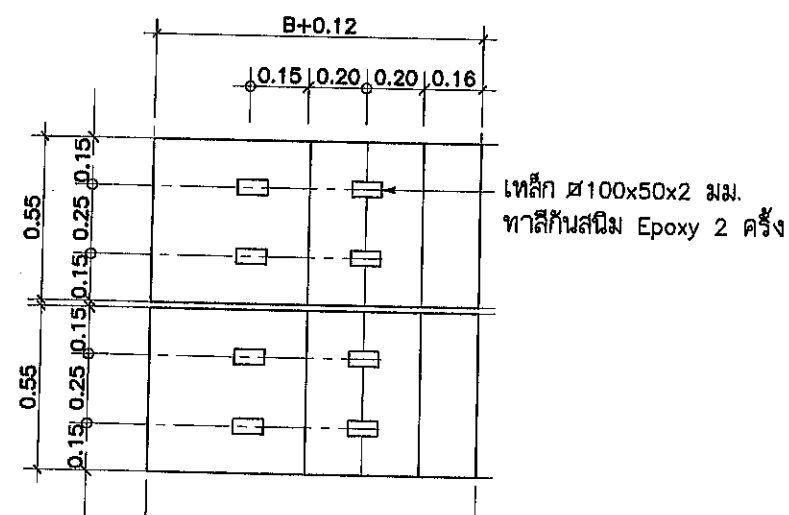
แปลนฝาข้อพับ ค.ส.ล.
