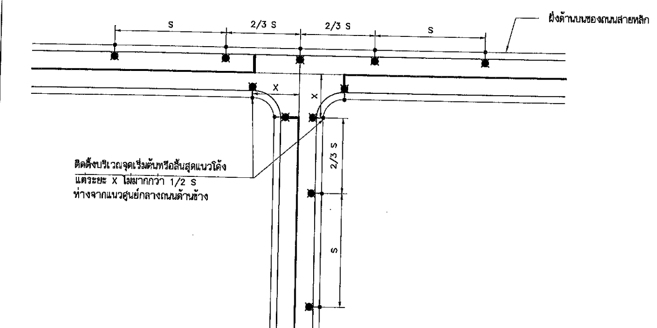
รูปแบบการติดตั้งเสาไฟฟ้าแสงสว่างถนนบริเวณสามแยก ไม่แสดงมาตราส่วน
