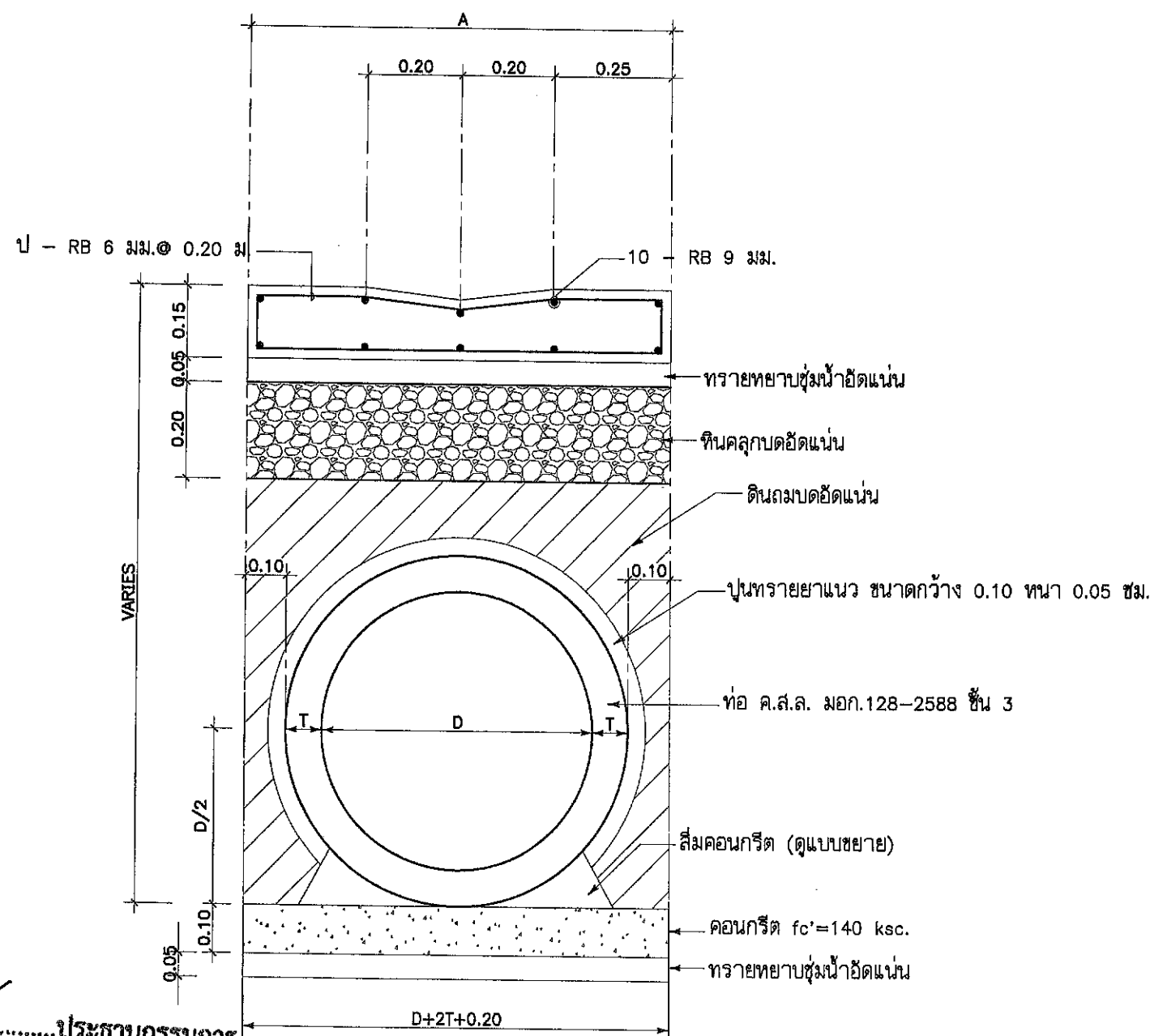
รูปตัด ⑤
