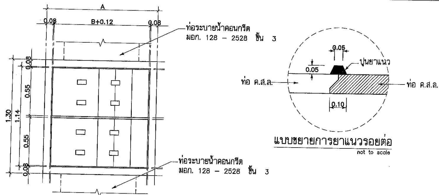
แปลนบ่อพัก ค.ส.ล.
