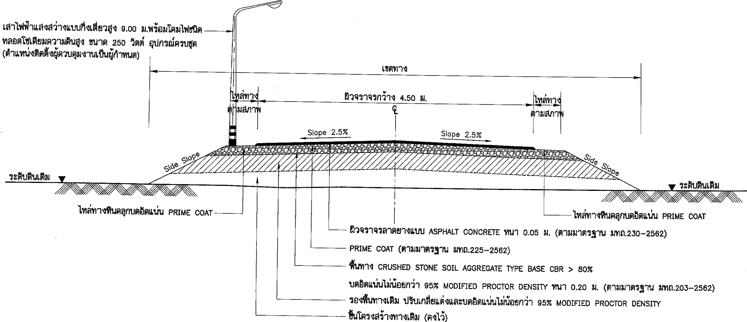
รูปตัดแสดงโครงสร้างถนนและคุณสมบัติวัสดุ (รูปตัดแสดงโครงสร้างชั้นทางเท่านั้น) (ช่วงที่ 1 Sta.0+242-Sta.0+362) NOT TO SCALE
